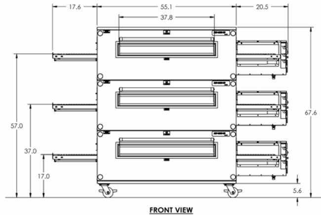
3255E-TS\TS2 & TS2E\TS2E Double and Triple Stack Model Dimensions
